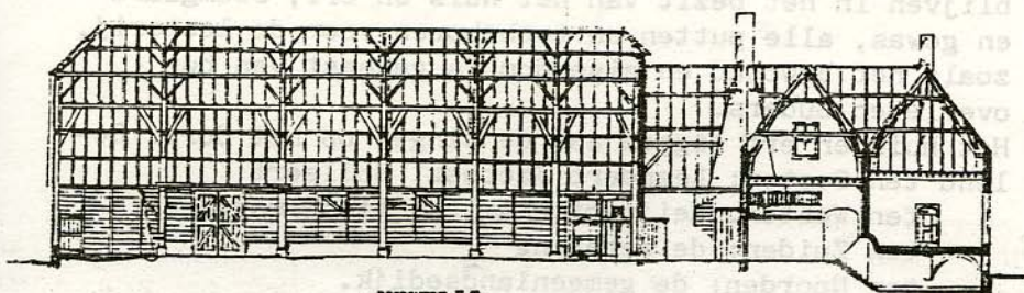
DOORSNEDEN E-F
