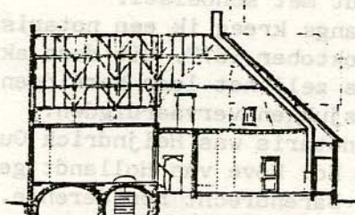
DOORSNEDEN A-B
